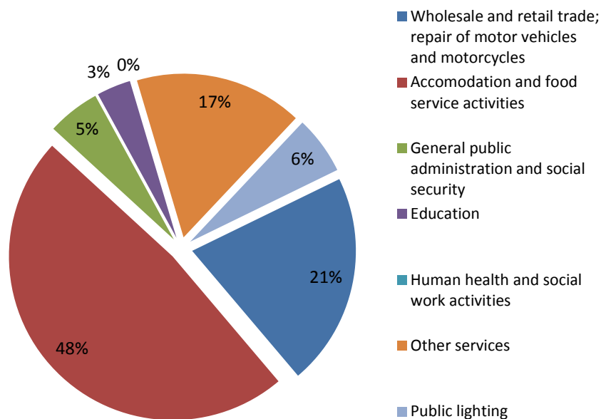
Διάγραμμα 3.6. Κατανομή της τελικής ζήτησης ενέργειας του τριτογενή τομέα στους υποτομείς
