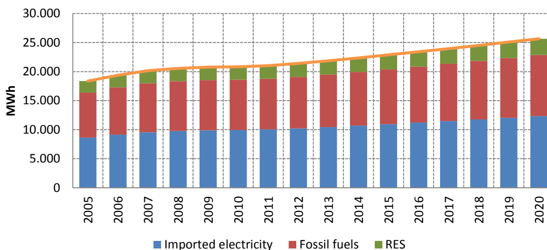
Διάγραμμα 3.19. BAU σενάριο – Τελική ζήτηση ενέργειας ανά ενεργειακή πηγή
