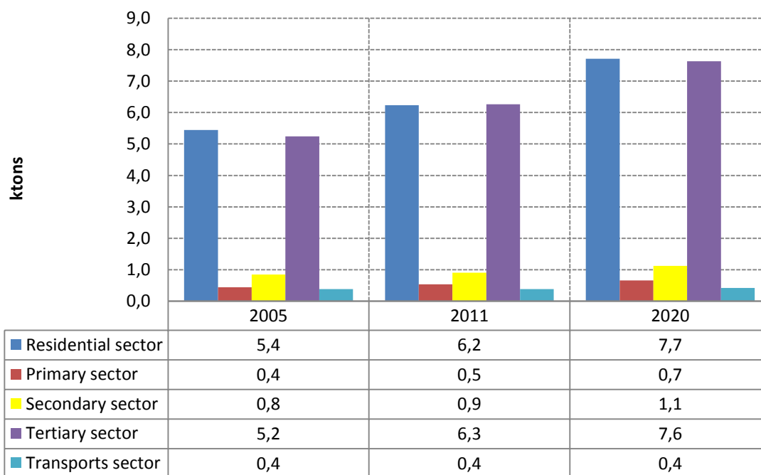
Διάγραμμα 3.28. BAU σενάριο – Προβολή εκπομπών CO 2 τελικής χρήσης ανά ενεργειακό φορέα
